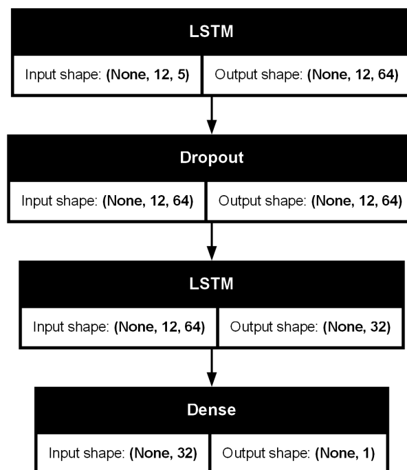
FIGURE 24 – Architecture du réseau de neurones avec couches LSTM utilisé.
