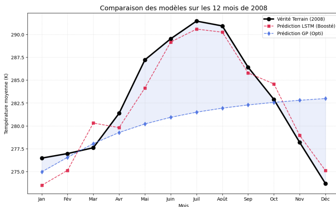
FIGURE 25 – Comparaison des modèles sur les 12 mois de 2008, l'année prédite.
