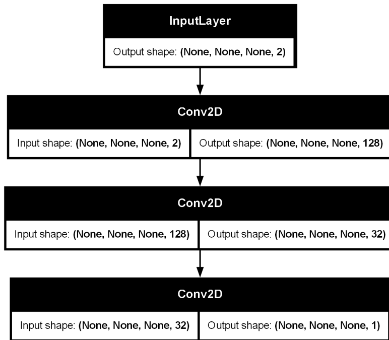
FIGURE 10 – Architecture CNN utilisé.
