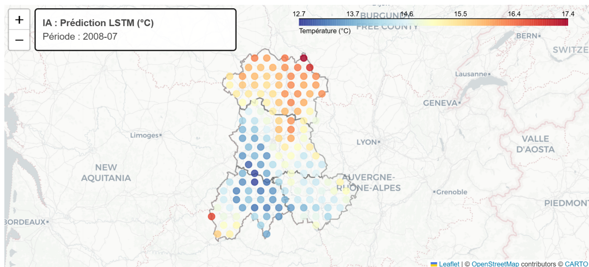
FIGURE 32 – Prédiction IA par réseau LSTM. On note la conservation des structures spatiales fines et la précision des gradients départementaux.
