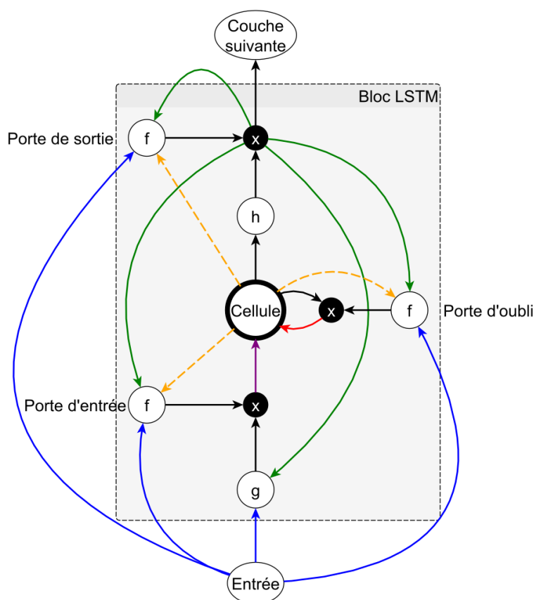
FIGURE 23 – Schéma d'un neurone LSTM comprenant une mémoire interne (cell) contrôlée par les trois portes d'entrée (input), d'oubli (forget) et de sortie (output). Schéma issu de la thèse de Bruno Stuner (2018). [13]
