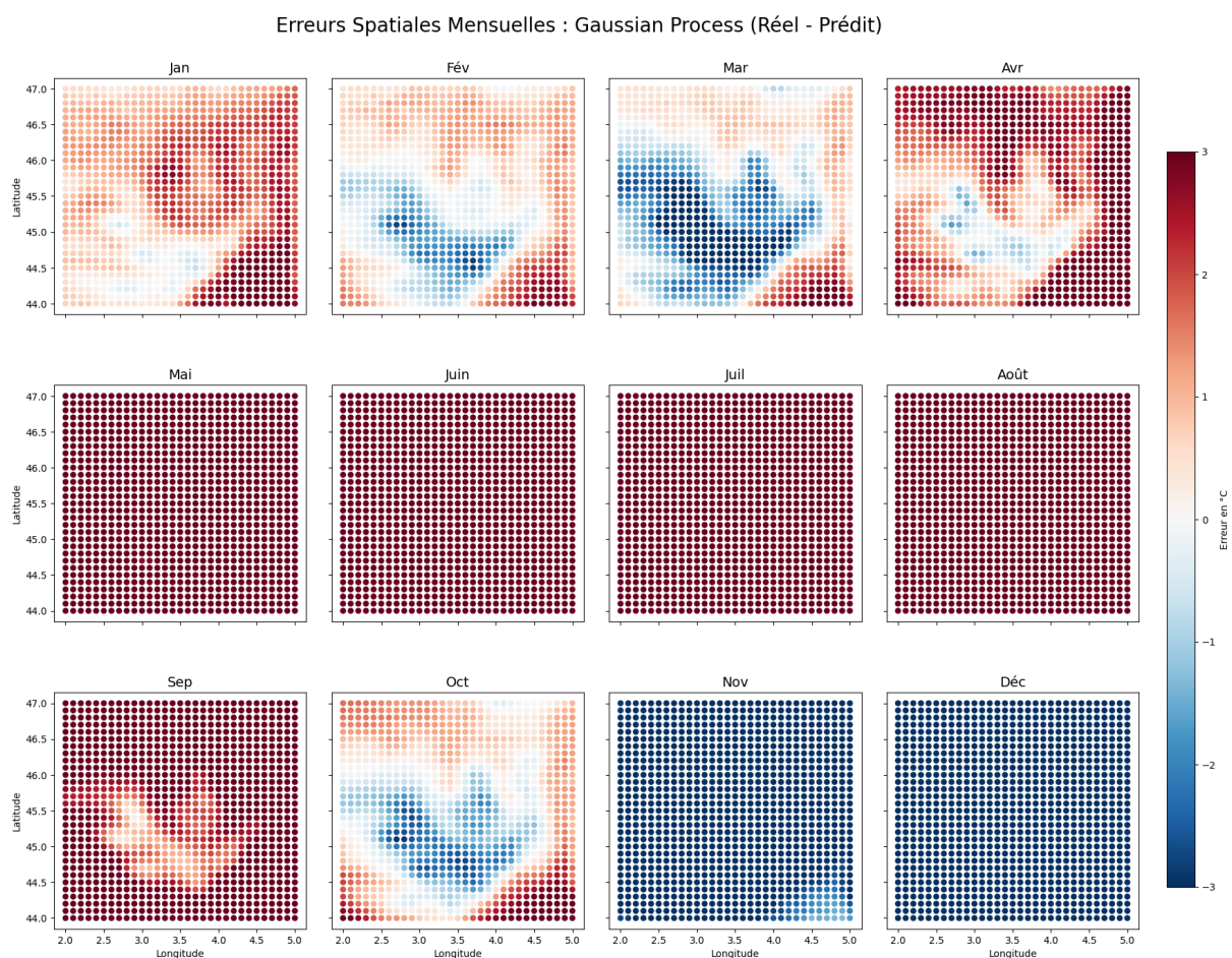
FIGURE 28 – Cartographie mensuelle des erreurs du modèle Gaussian Process (GP).
