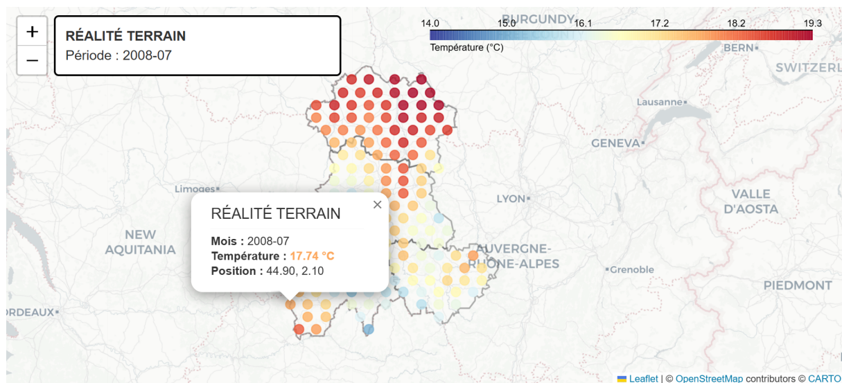
FIGURE 31 – Réalité terrain ERA5-Land pour juillet 2008. La palette de couleurs illustre le gradient thermique naturel lié au relief auvergnat.
