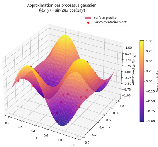
FIGURE 11 – Prédiction GP capturant les extrema de la fonction f_2 .
